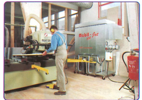
Mobil-Jet 200 als dezentrale Absauglösung z.B. für eine CNC-Oberfräse.
