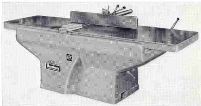
Schwere Abrichthobel-, Füge-, Kehl- und Falzmaschine Modell DA 41/51/63, Arbeitsbreite 410, 510 und 630 mm
