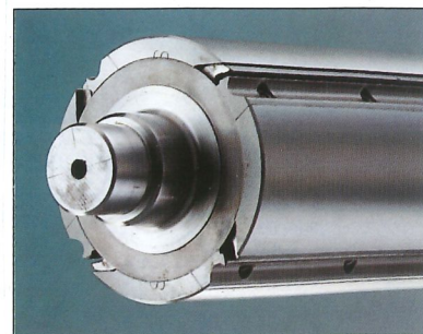
Albero pialla "MONOBLOC" con coltelli Tersa Planer shaft "MONOBLOC" with Tersa knives Arbre "MONOBLOC" avec couteaux Tersa "MONOBLOC"-Messerhobelwelle mit TERSA- Messern Eje "MONOBLOC" con cuchillas Tersa
