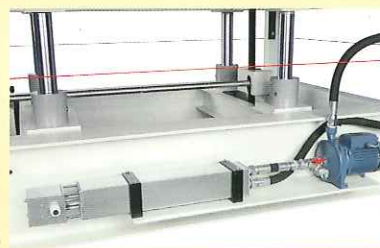
Heizung bei der Ausführung mit Stahlheizplatten
