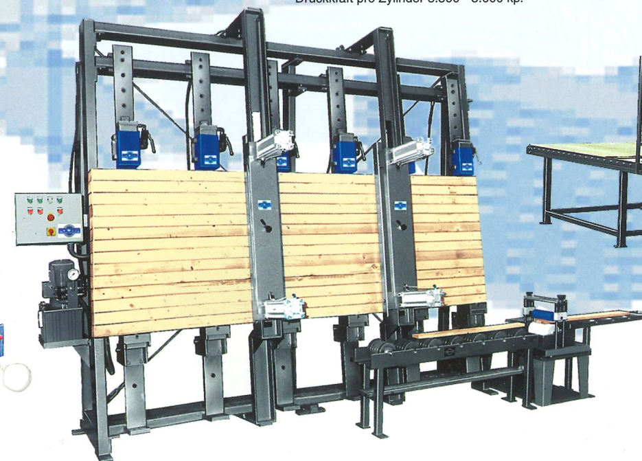
Elektro-Hydraulik-Kompakt-Block- und Lamellierpresse, Druckkraft pro Zylinder 3.500 - 5.000 kp.
