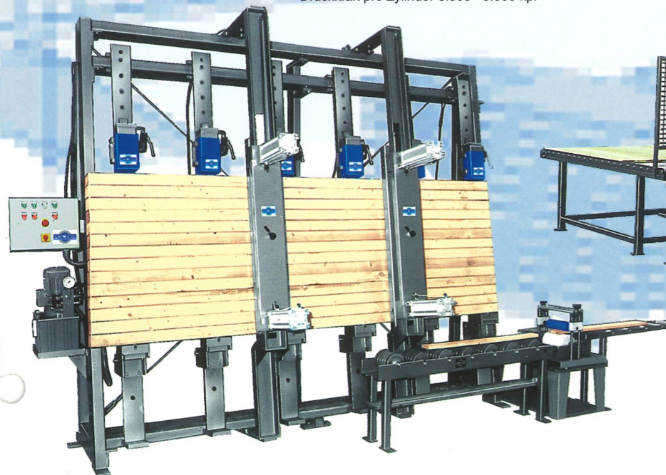
Elektro-Hydraulik-Kompakt-Block- und Lamellierpresse, Druckkraft pro Zylinder 3.500 - 5.000 kp.
