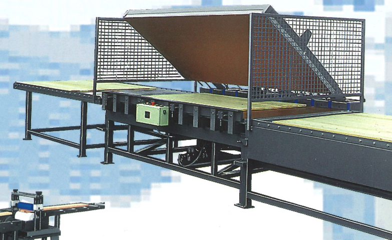
Beheizte Etagen-Verleimstation mit Ein- und Ausschubvorrichtung.
