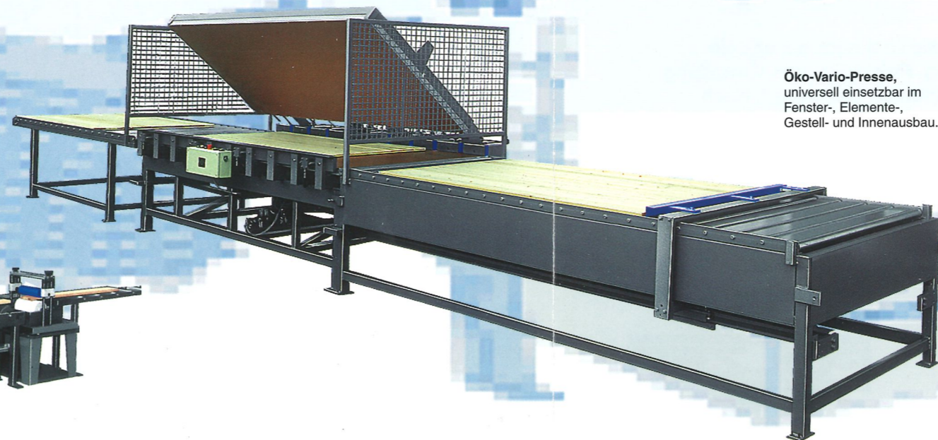
Beheizte Etagen-Verleimstation mit Ein- und Ausschubvorrichtung.
