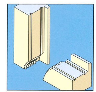
◀ Kreisbogen CNC Eckverbindung Genius®
